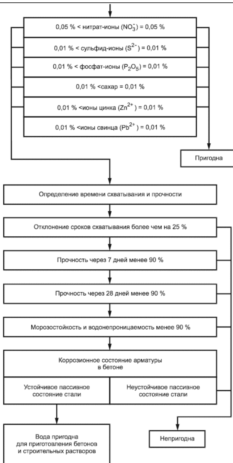
Рисунок А.1 (лист 2)
